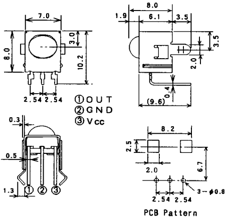
NJL57H000 UNIT : mm
