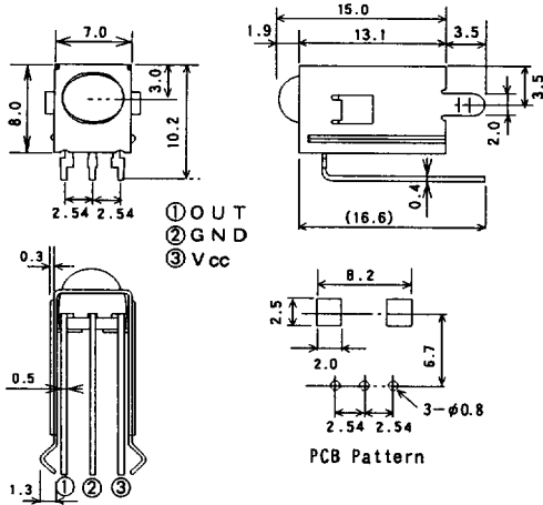
NJL56H000 UNIT : mm
